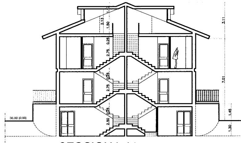
SECCION b-b'
